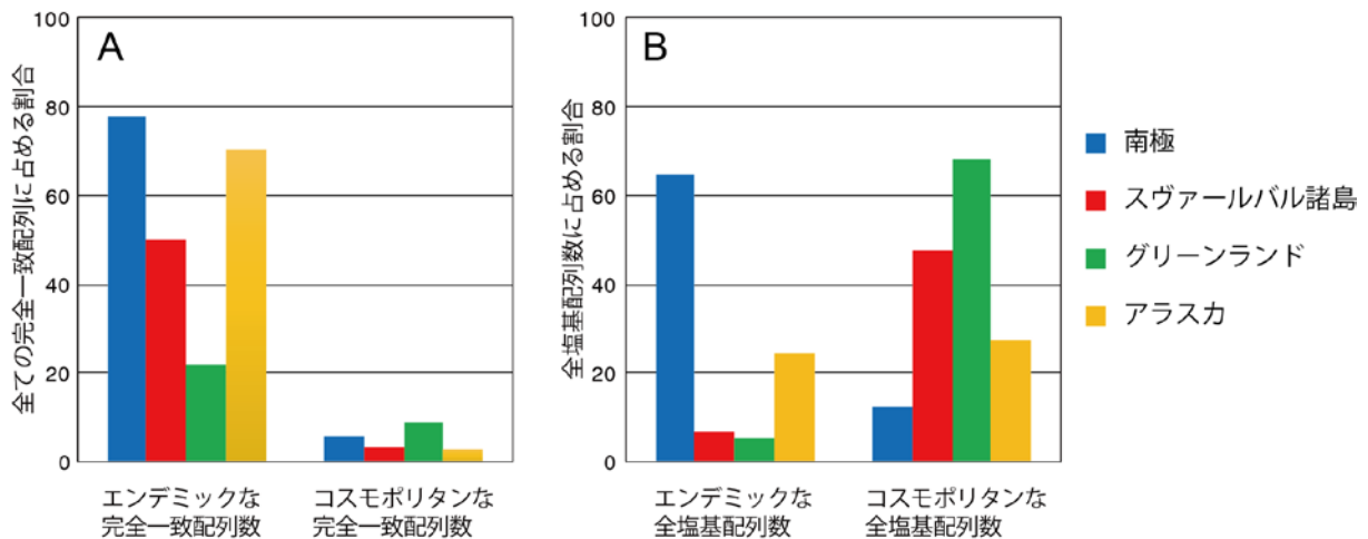
図4 両極から検出された雪氷藻類の割合
