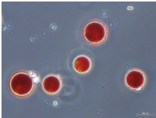
赤い色素をもった雪氷藻類の増殖により，雪が赤く染まる.
