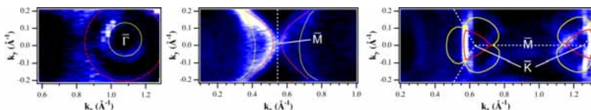
図5 点、M点、K点まわりの等エネルギー面
