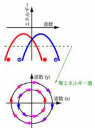
図1 ラシュバ効果による電子バンドの分裂と等エネルギー面
