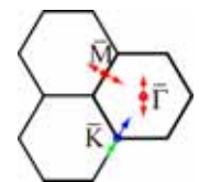
図4 時間反転
