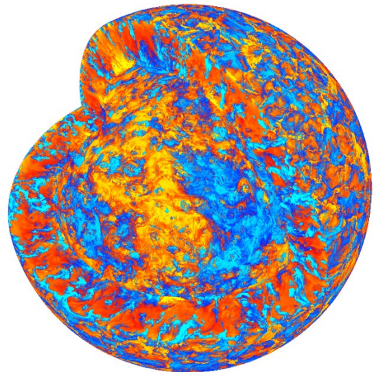
「富岳」で再現された太陽内部熱対流の様子。熱対流を表現するのに適したエントロピーという量を示しています。橙、青の部分はそれぞれ暖かい・冷たい領域に対応します。
