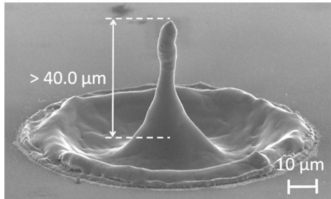
▲図1 シリコンニードル (照射エネルギー0.6 mJ/pulse、照射パルス数12)
