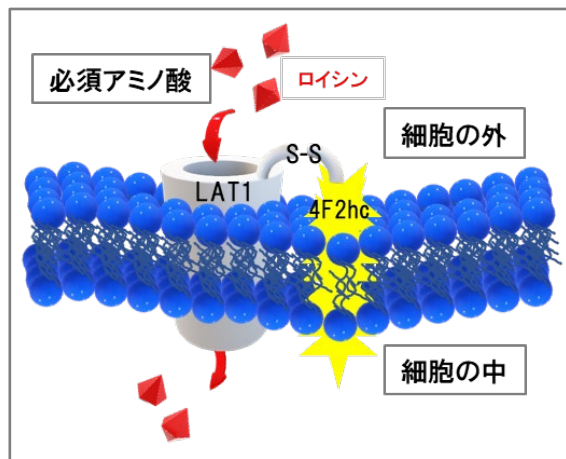
図 1 LAT1-4F2hc の模式図。がん細胞の中に必須アミノ酸を運ぶ役割をしている。
