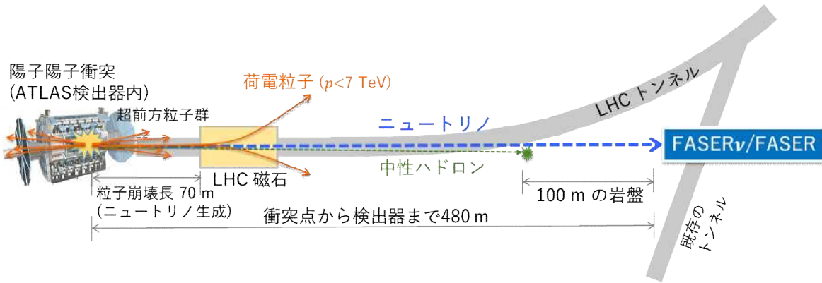
図 1. LHC の陽子陽子衝突点と FASERν 検出器の設置位置
