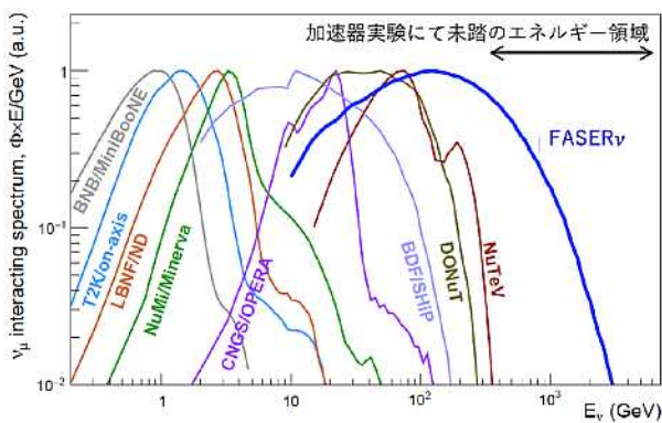
図 2. FASERν で測定予定のエネルギー領域 (濃い青い線) と先行研究で測定されてきたエネルギー領域 (その他の色の線)。横軸はニュートリノのエネルギー、縦軸は 1 GeV あたりのニュートリノ反応数 (最大値が 1 になるように規格化したもの) を示しています。FASERν は黒い矢印で示した高エネルギー領域で加速器実験として史上初の測定を行います。
