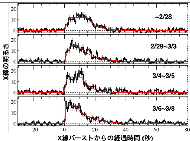
図 5 NinjaSat が観測した SRGA J1444 からの X 線バーストの特徴
