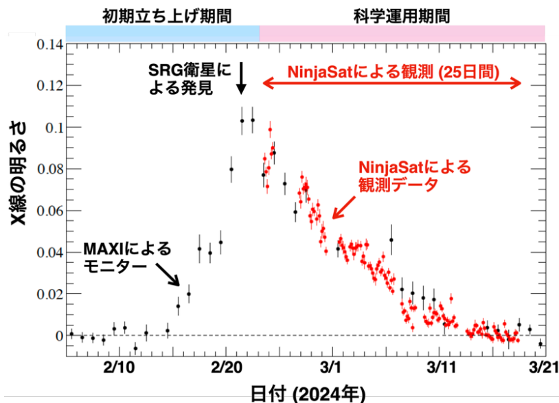
図 3 NinjaSat が観測した SRGA J1444 の X 線強度変化
